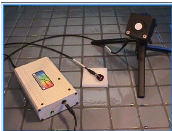
شکل ۱۴- نمونه دستگاه اسپکترو رادیومتر فرابنفش
